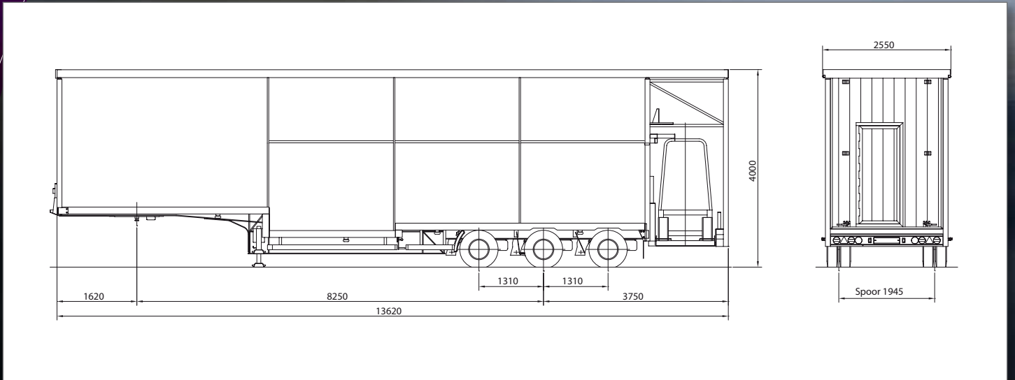
Heineken laad- en lossysteem voorzien van kettingbanen.
